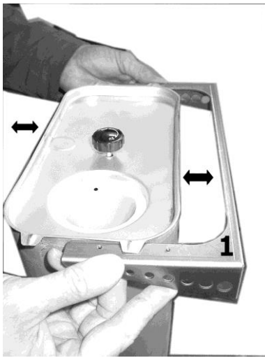
Abbildung 3: Montage des Tankbügels 1 Tankbügel
