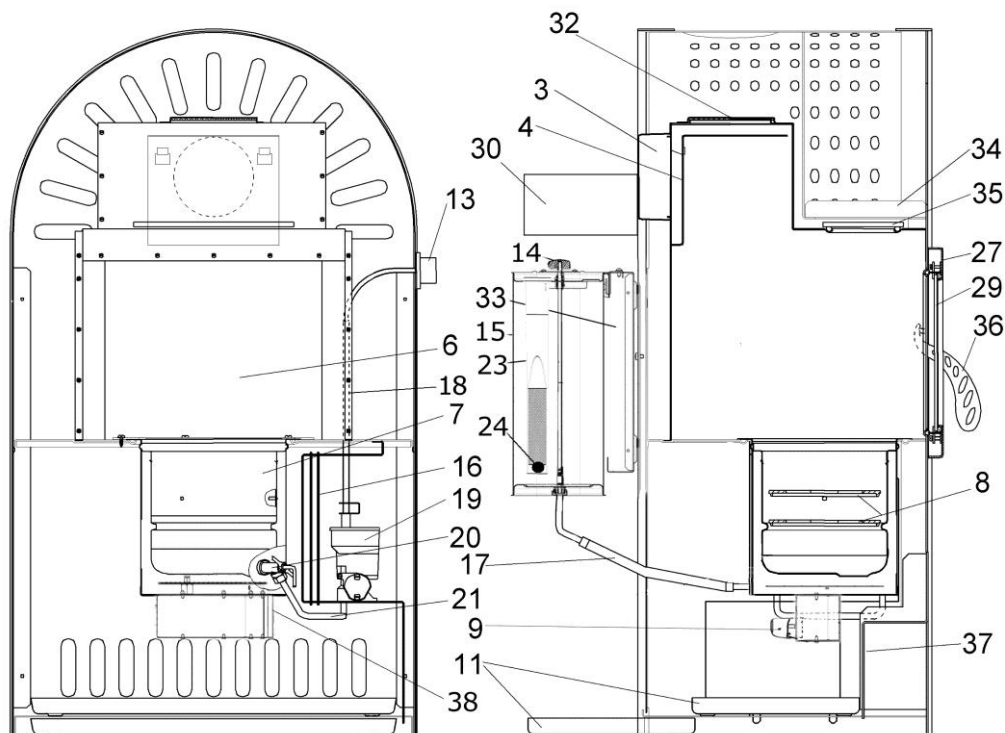
Abbildung 1: Ölofen Viking 468.50
