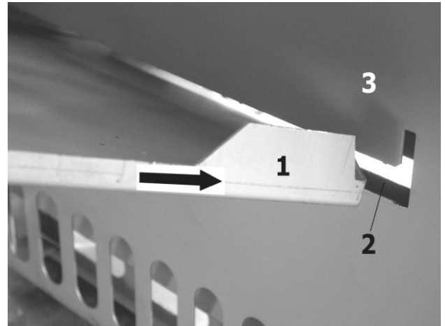
Abbildung 11: Ibiza 469.50, Montage des Ölleitblech
