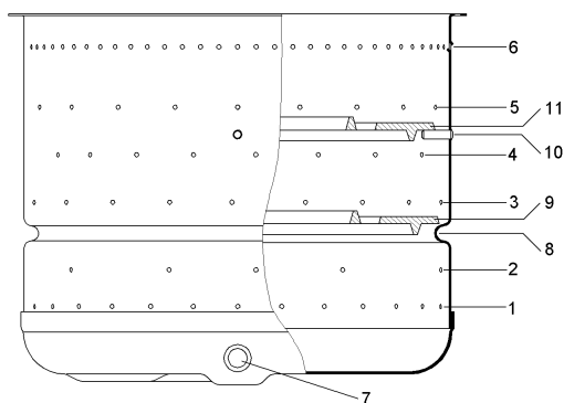
Abbildung 18: Brenner mit Brennerringe
