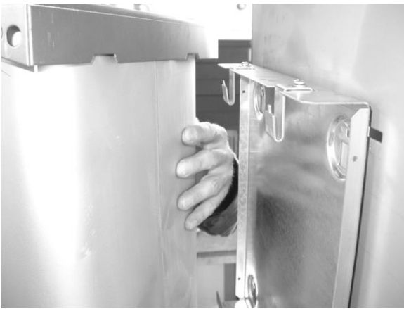
Abbildung 9: Montage des Öltanks
