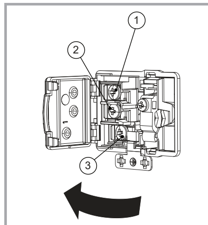
Abb. 17 - Klemmbrett für den Anschluss die Stromversorgung: 1. Phase, 2. Neutralleiter, 3. Schutzleiter.
