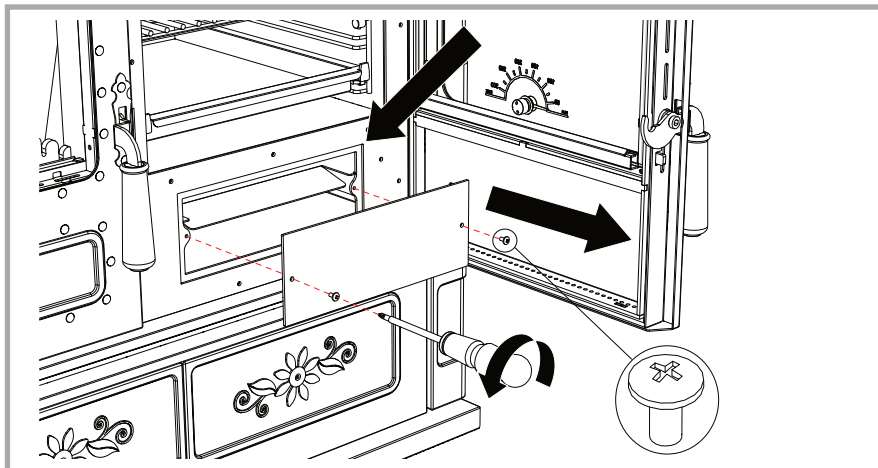
Figura 36 – Ispezione girofumi.
