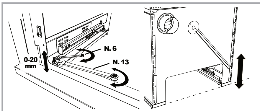
Figura 15 – Regolazione dell'altezza dell'apparecchio mediante i piedini livellatori con chiave esagonale.
