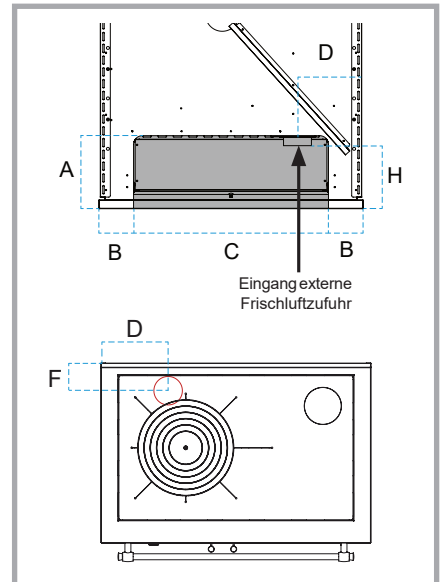
Abb. 13 – Hinteransicht des Sockels und Angaben für den Anschluss die externe Frischluftzufuhr.
