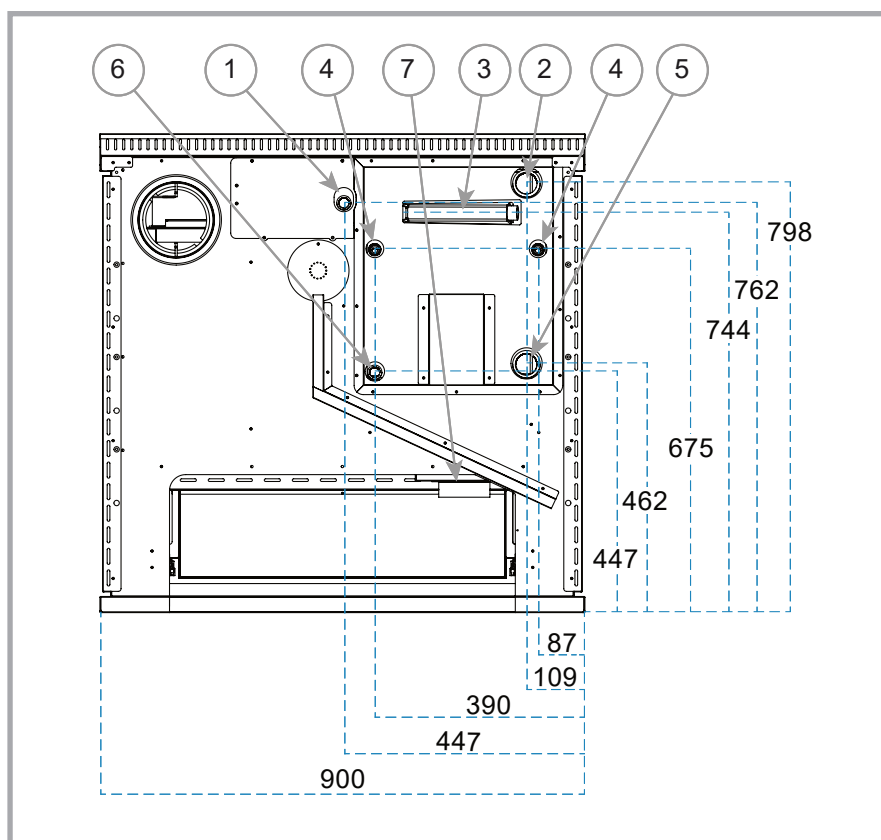
Abb. 19 - Anschlussschemades Modells LT 90 mit Rauchausgang rechts (Rückansicht). Beim Modell mit Rauchausgang links befinden sich die Anschlüsse symmetrisch.
