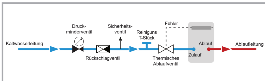
Abb. 20 – Schematische Darstellung für den Kreislauf des Sicherheitswärmetauschers.
