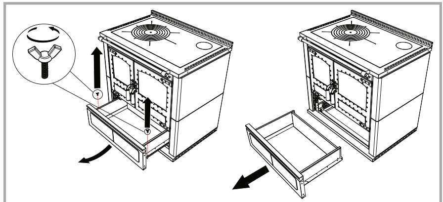
Abb. 14 - Entfernung der Holzlade.
