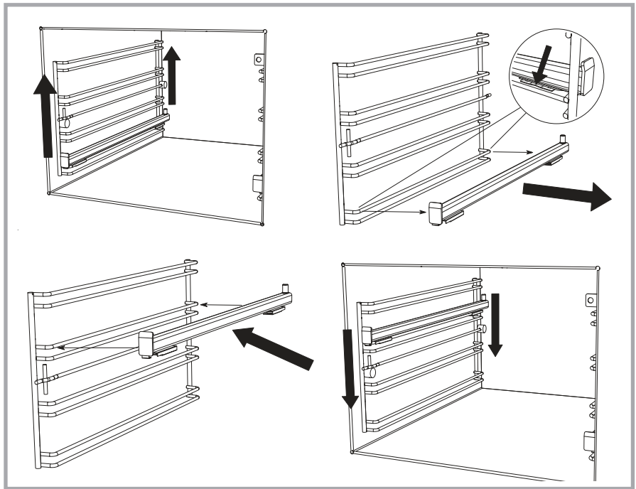
Abb. 32 – Vorgangsweise zum Umstecken des Teleskopauszugs.
