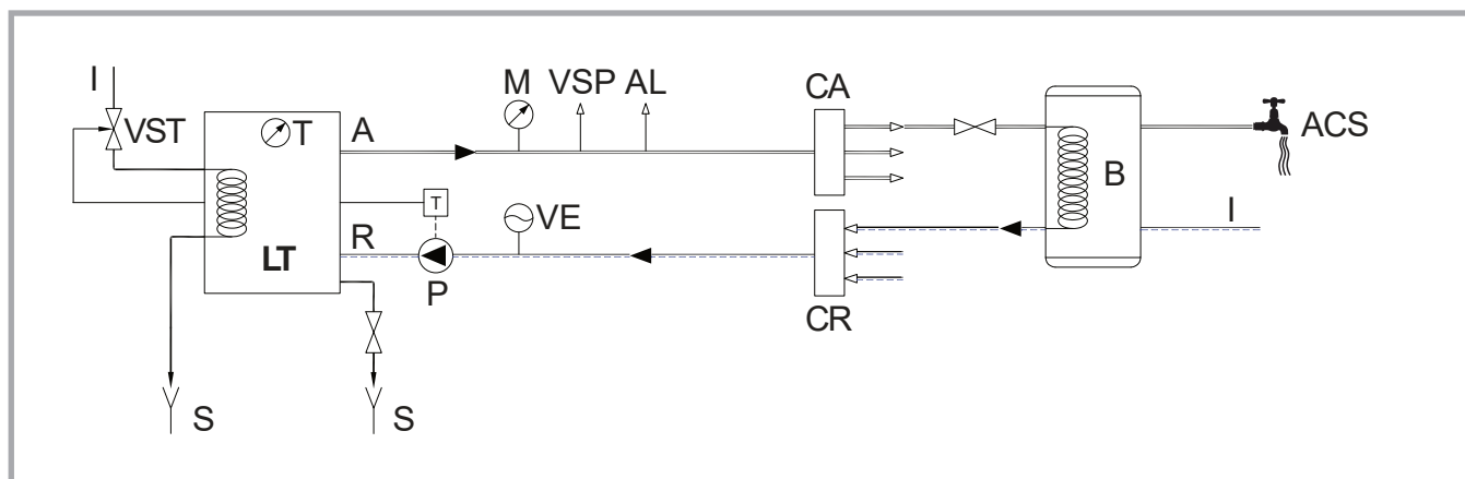
Abb. 21 – Schematische Darstellung zur Realisierung einer Heizungsanlage mit einem Zentralheizungsherd LT 90 als Wärmeerzeuger.
