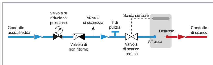
Figura 20 – Schemarealizzativo del circuito di scarico termico.
