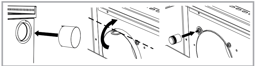
Abb. 9 - Rauchausgangseitlich. Befestigung des Anschlussrohrs bei seitlichem Rauchausgang.
