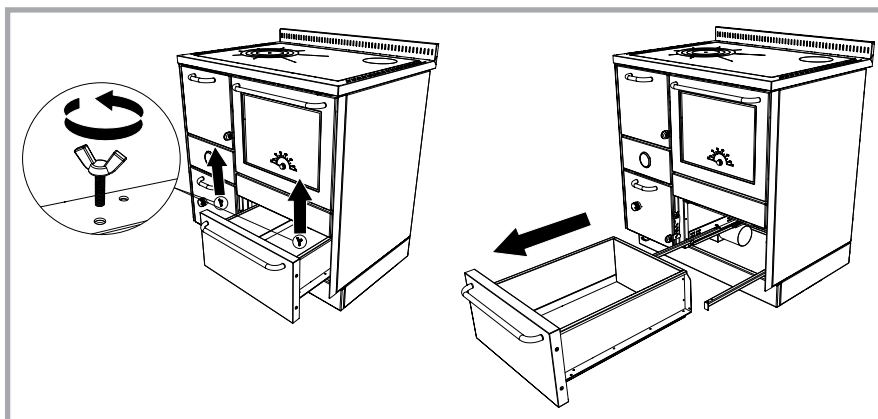
Figura 17 – Estrazione cassa porta legna.
