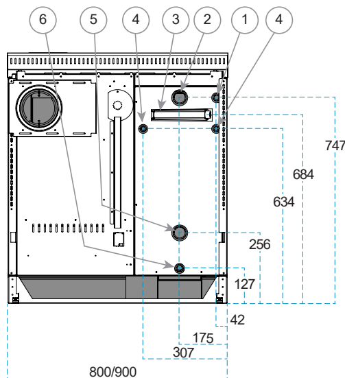
Abb. 21 - Anschlussschemader Modelle RTE 80, RTVE 80, RTE 90 und RTVE 90 mit Rauchausgangrechts (Rückansicht). Bei Modellen mit Rauchausganglinks befinden sich die Anschlüsse symmetrisch.
