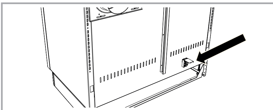
Figura 15 – Posizione della morsetteria per l'allacciamento alla rete elettrica.
