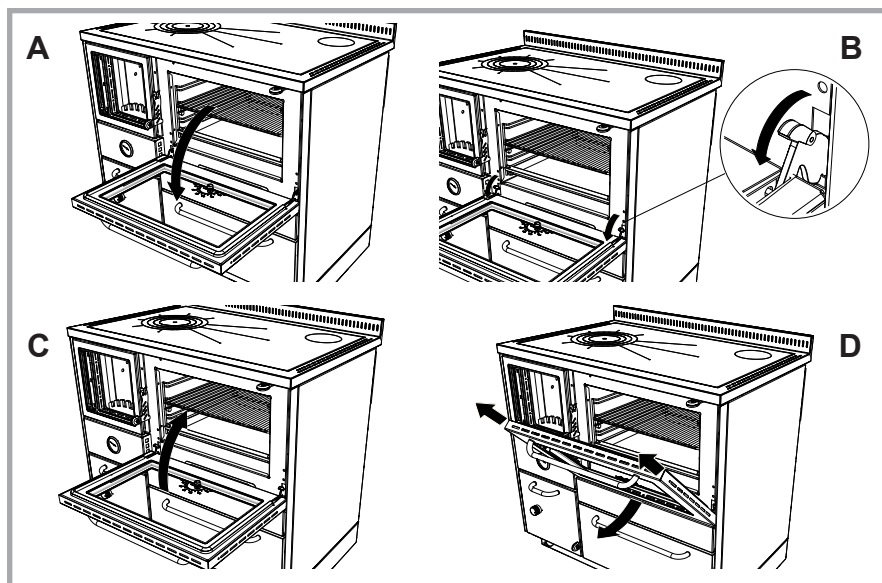
Abb. 41 - Aushängender Backofentür.
