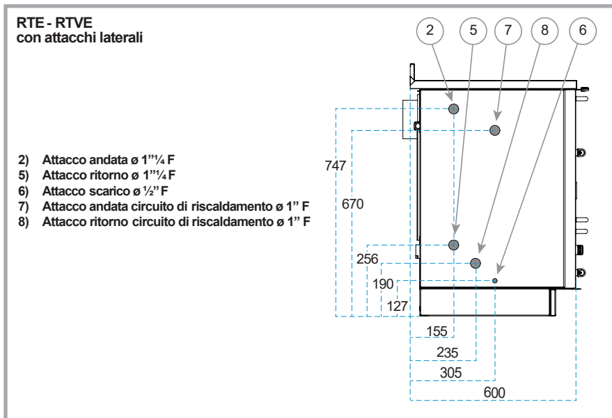
Figura 22 – Posizione degli attacchi caldaia per i modelli RTE/RTVE con attacchi laterali (vista laterale).
