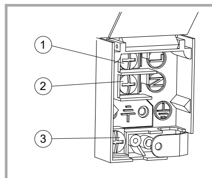
Figura 16 – Morsetteria elettrica per il collegamento alla rete: 1. Linea 2. Neutro 3. Terra
