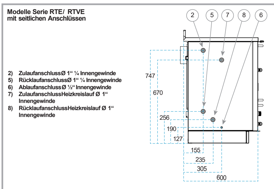
Abb. 22 - Anschlussschemader Modelle RTE/ RTVE mit seitlichen Anschlüssen(Seitenansicht).
