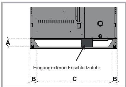
Abb. 14 - Rückansicht des Sockels und Angaben für den Anschluss der externen Frischluftzufuhr.
