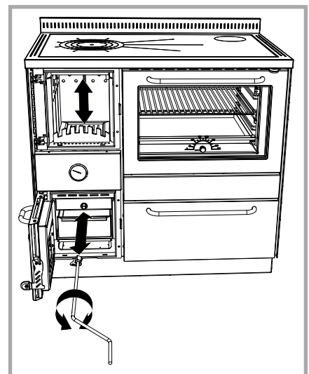
Abb. 32 - Höhenverstellbarer Feuerrost
