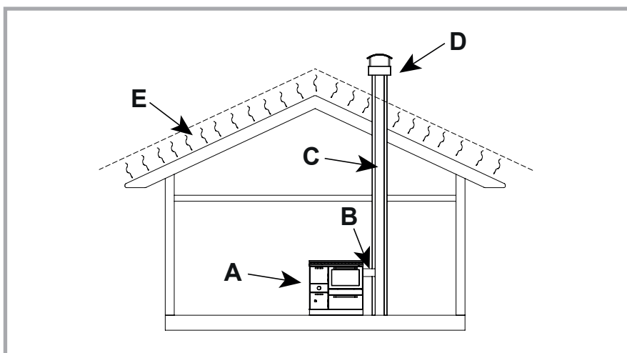
Abb. 3 - Teile des Kamins A = Zentralheizungsherd, B = Rauchrohrstützen, C = Rauchabzug, D = Schornstein, E = Windfangbereich
