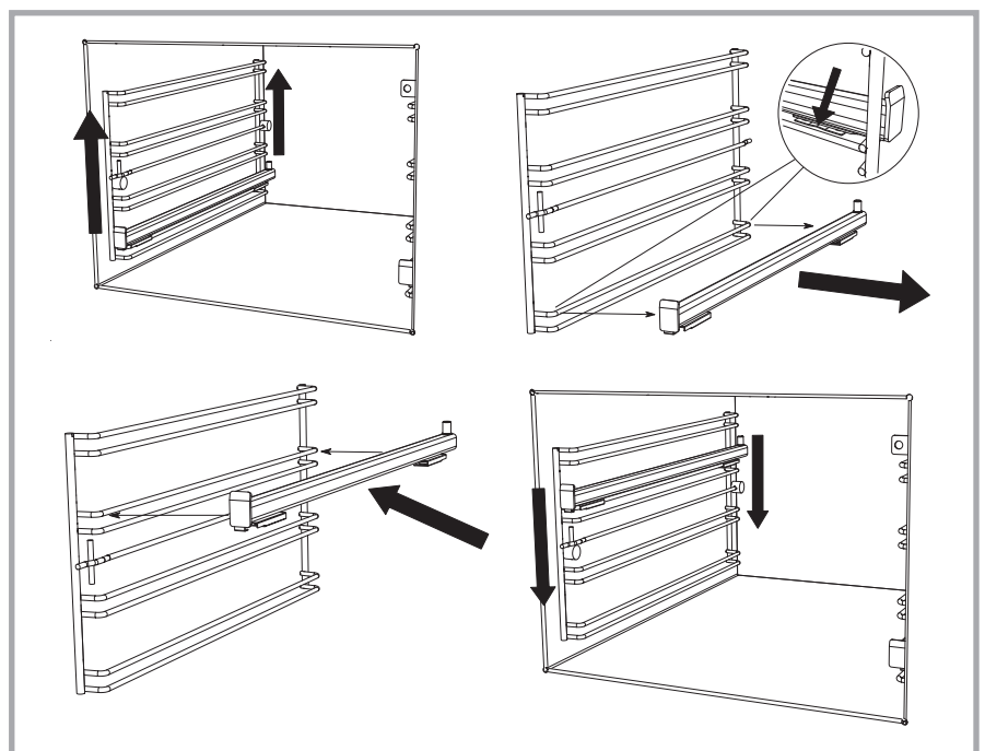
Abb. 34 - Vorgangsweise zum Umstecken des Teleskopauszugs.
