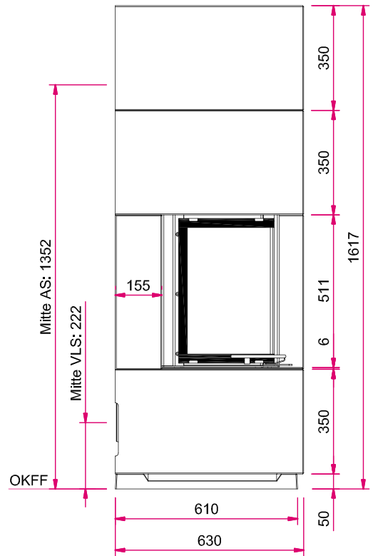
Seitenansicht
