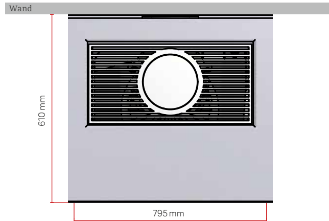
Estrichaussparung
