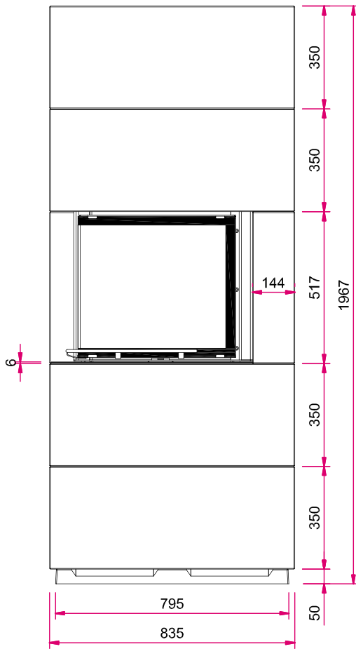
Frontansicht
