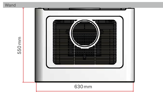
Estrichaussparung
