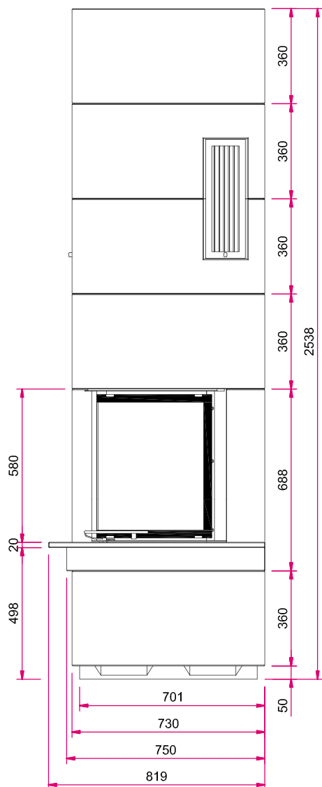
Frontansicht M 1:20
