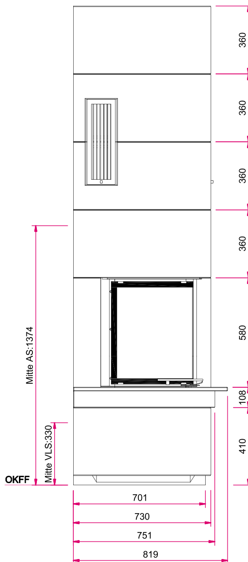
Seitenansicht links M 1:20
