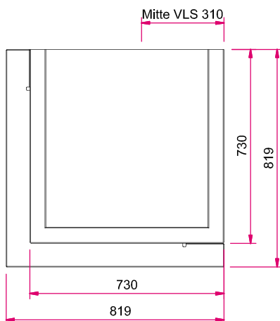
Draufsicht M 1:20
