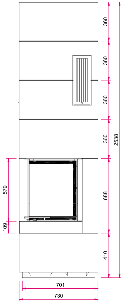
Frontansicht M 1:20
