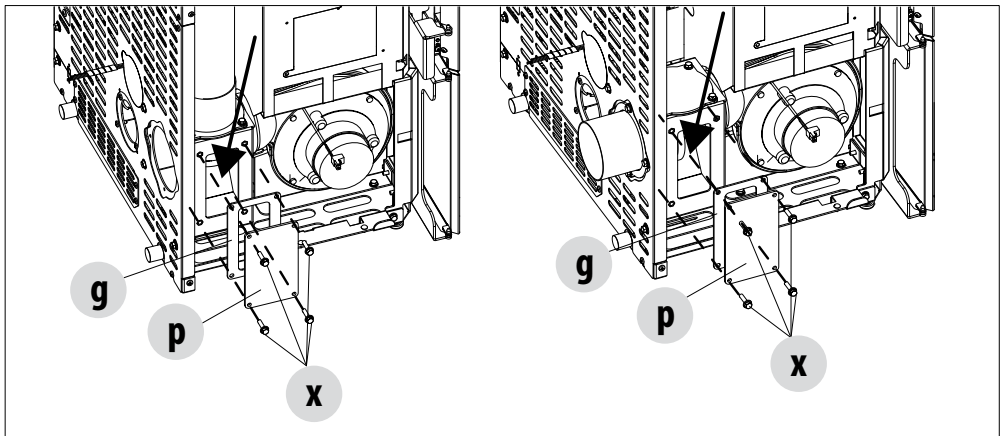
REINIGUNG RAUCHGASABZUG OBEN
