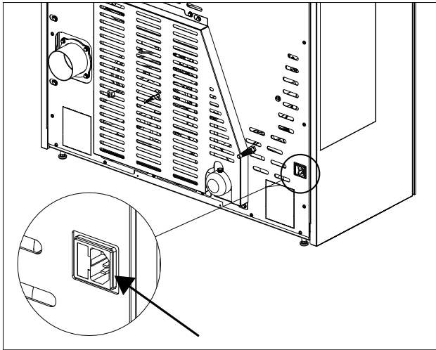
ELEKTRISCHER ANSCHLUSS DES OFENS.
