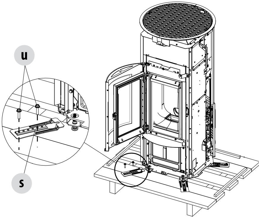
ENTFERNUNG DER BEFESTIGUNGSWINKEL OFEN MOOD
