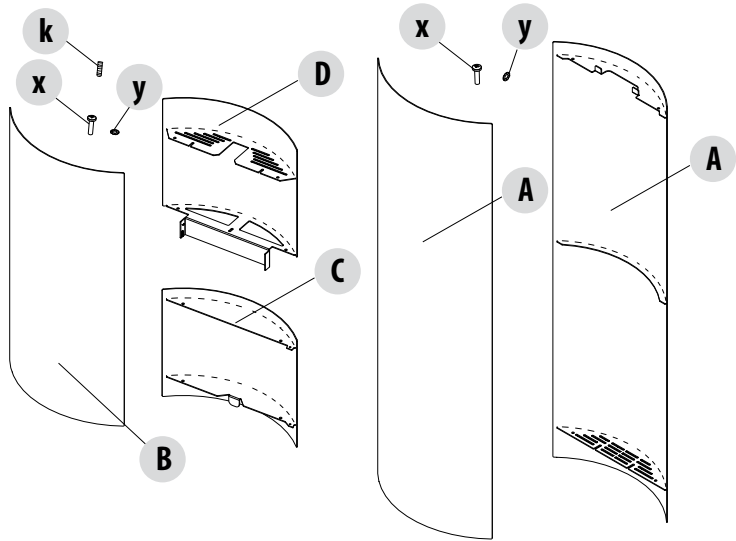
METALLVERKLEIDUNG
